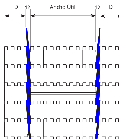
MEDIDAS ESTÁNDARES DE “D”[mm]
