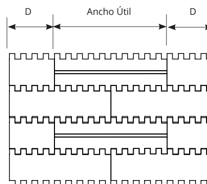
MEDIDAS ESTÁNDARES DE “D”[mm]
