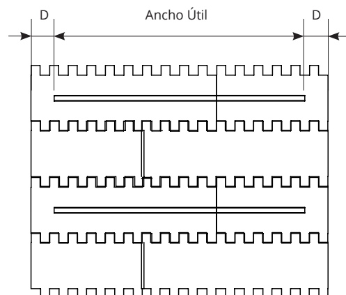
MEDIDAS ESTÁNDARES DE “D”[mm]
